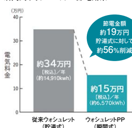
瞬間式ウォシュレットの節電効果
