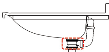
<MLHC (オーバーフローあり) 側面図>
