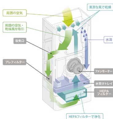
本体構造イメージ図
