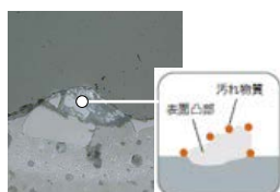
従来タイル(※1)(特殊加工なし) ※1 MBシリーズ
