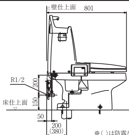
側面図
