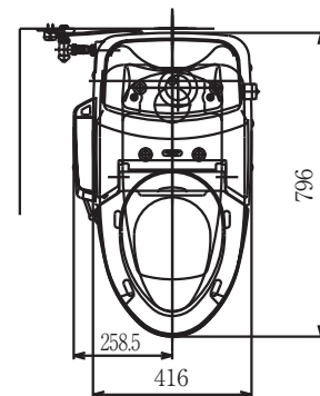
平面図
