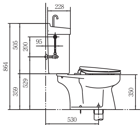
側面図
