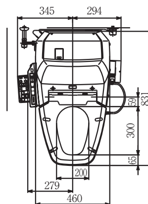
平面図
