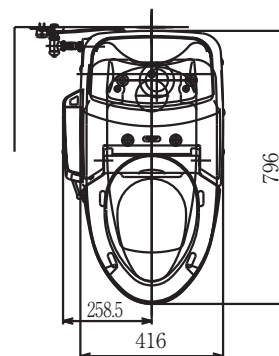
平面図
