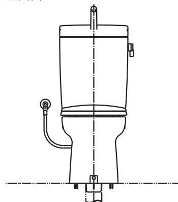
正面図
