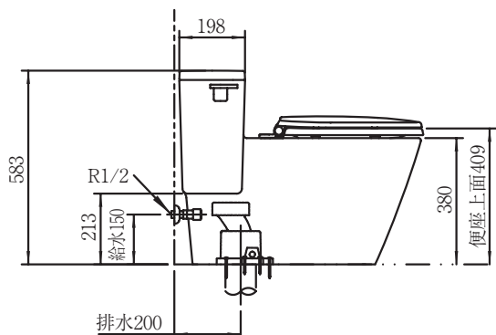
側面図
