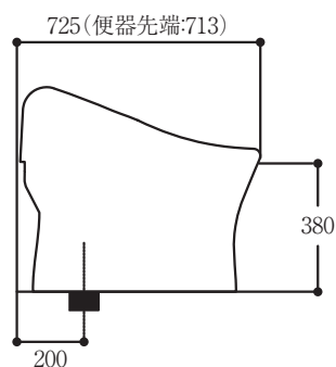
側面図
