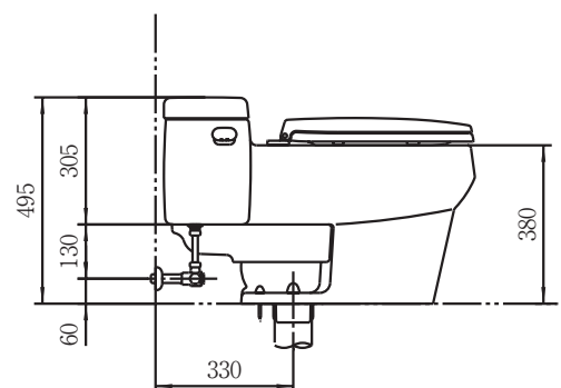
側面図
