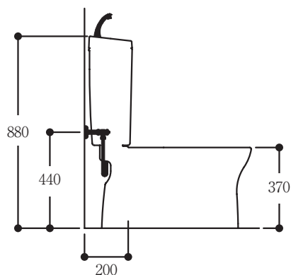
側面図
