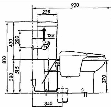
側面図
