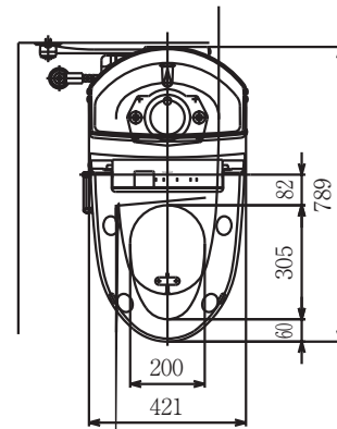
平面図
