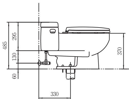
側面図
