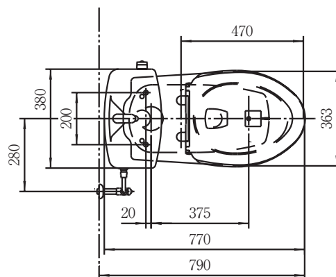
平面図
