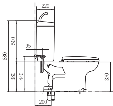
側面図
