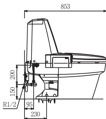
側面図
