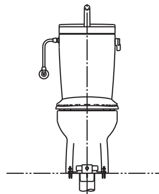
正面図
