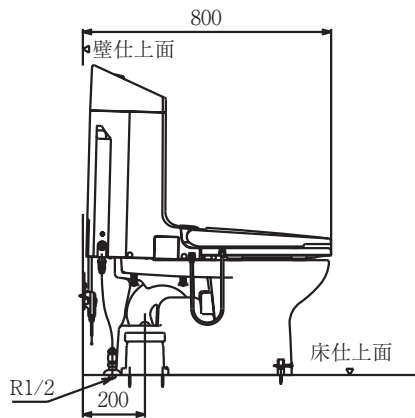
側面図
