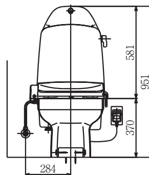
正面図
