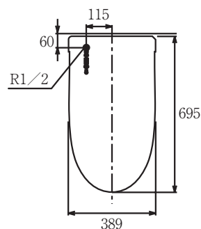
平面図
