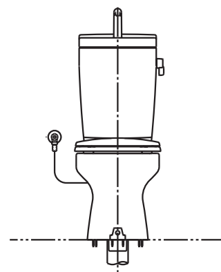
正面図
