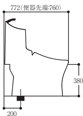
側面図
