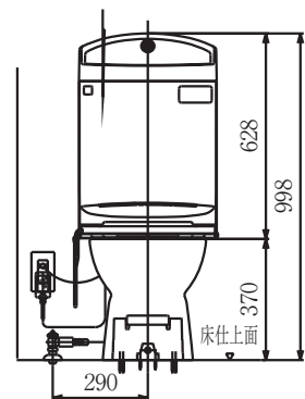
正面図
