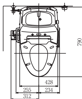
平面図
