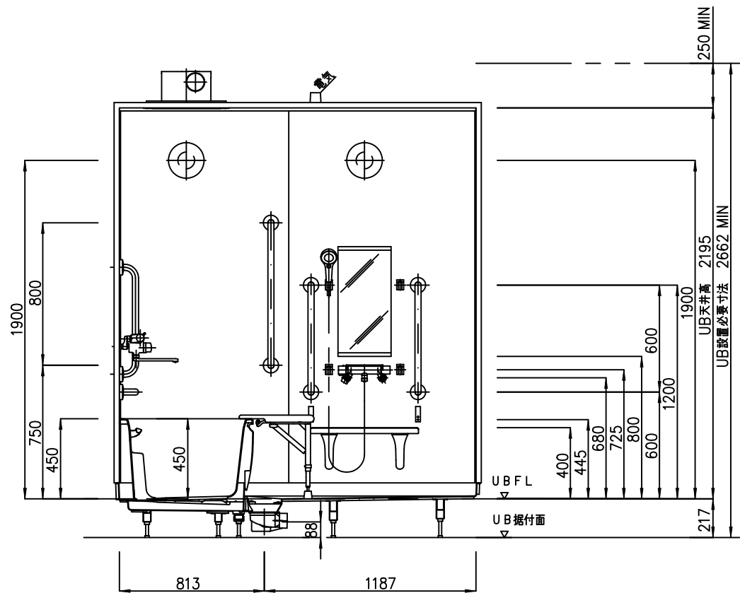
( ) 寸法は床のドア下部分を含む寸法
