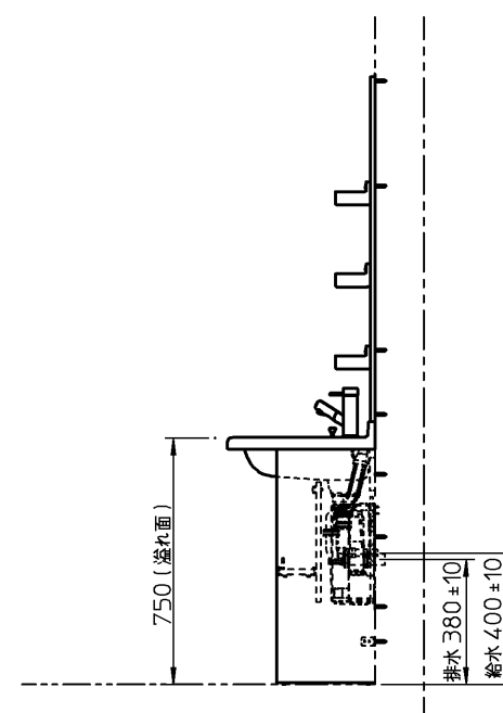
マープライトカウンタ側面図
