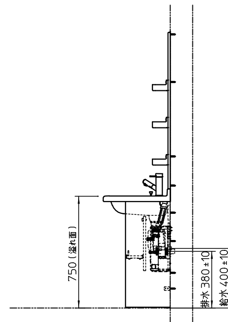
マーブライトカウンター側面図
