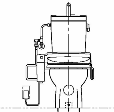
正面図
