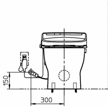
正面図
