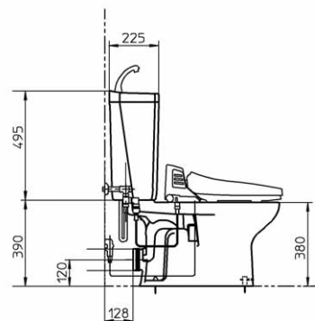
側面図
