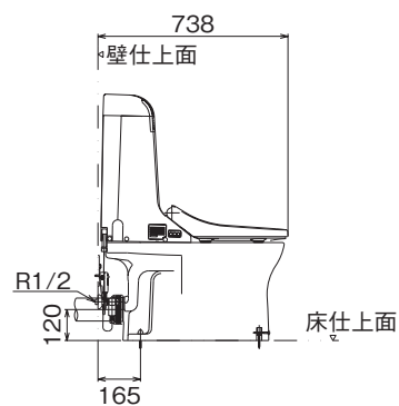
側面図
