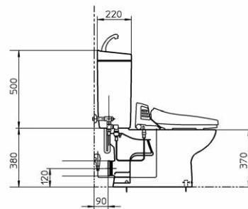
側面図
