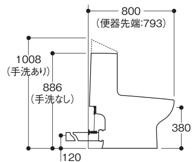
側面図
