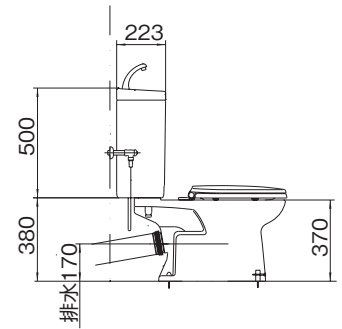
側面図
