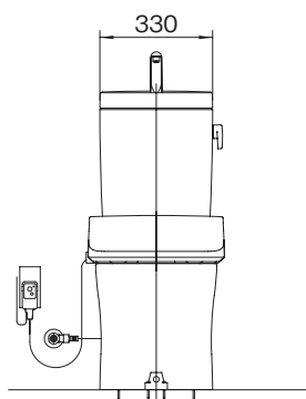
正面図
