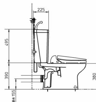
側面図
