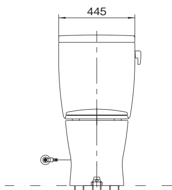
正面図
