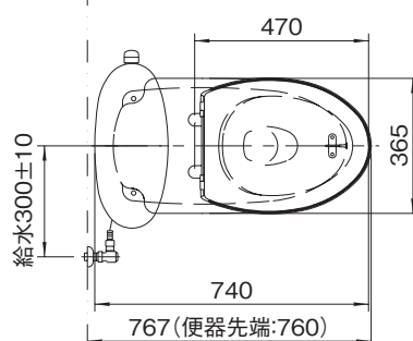
平面図
