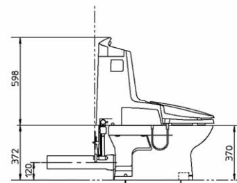
側面図
