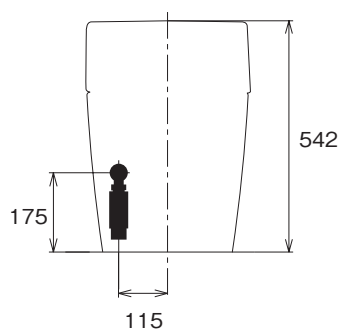
正面図
