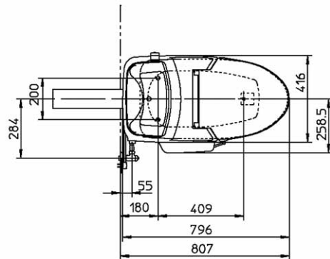
平面図
