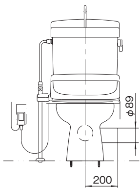
正面図
