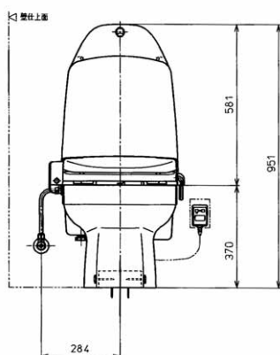
正面図
