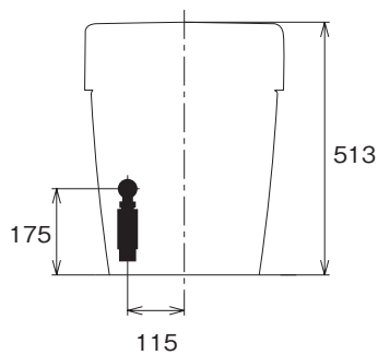
正面図
