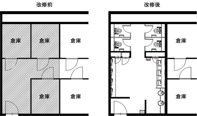
トイレ図面
