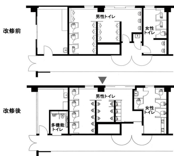
トイレ図面
