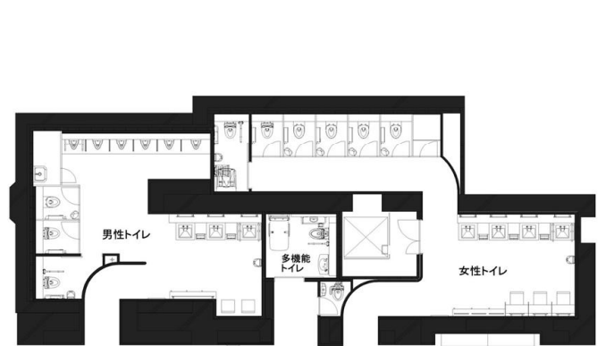
トイレ図面
