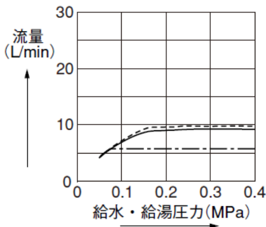
エアインシャワー TMN 40TE型・TE 3型
