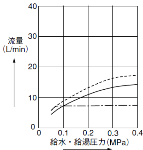
エアインシャワー TMWB 40EC型
