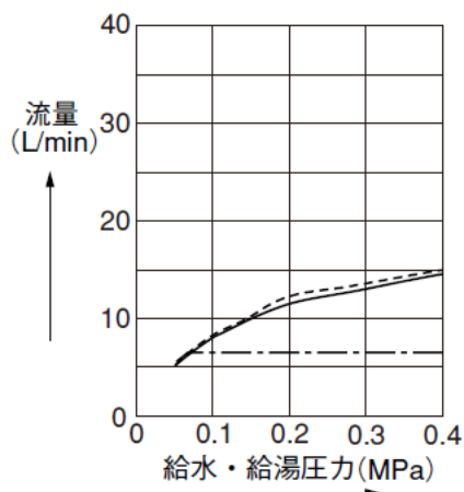
エアインシャワー TMF 44E型
