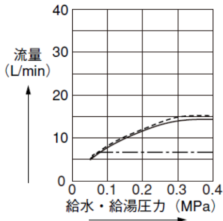
エアインシャワー TMF 49E型
