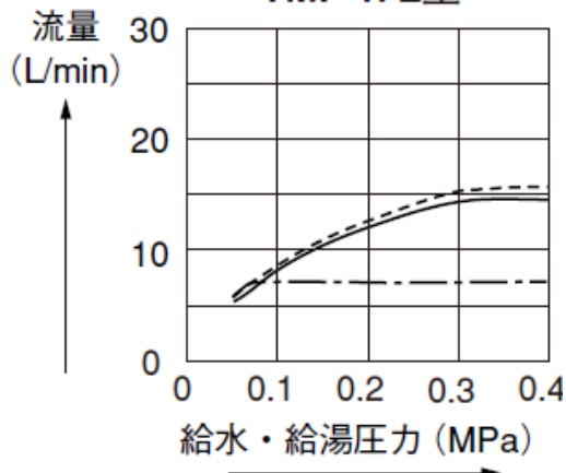
エアインシャワー TMF 47E型
