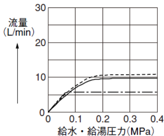
エアインシャワー TMN 40TEC型
