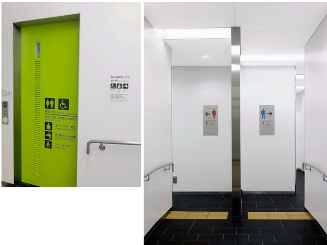
手前に「みんなのトイレ」入口、奥に男女トイレ入口がある。入口に続く通路は緩やかなスロープになっている。
