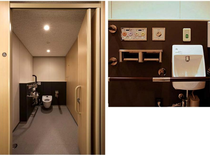
車いす使用者に配慮して、大便器ブースの1ヶ所には、ブース内に手洗器を設置した、個室完結型のひろびろブースを設けている。
