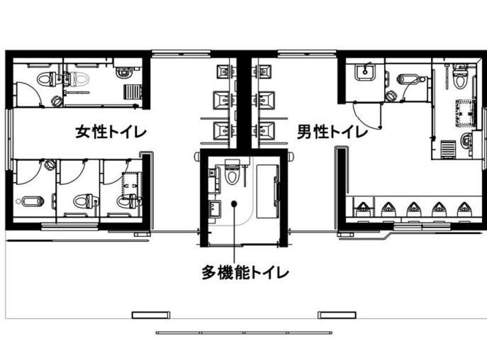
トイレ 図面
